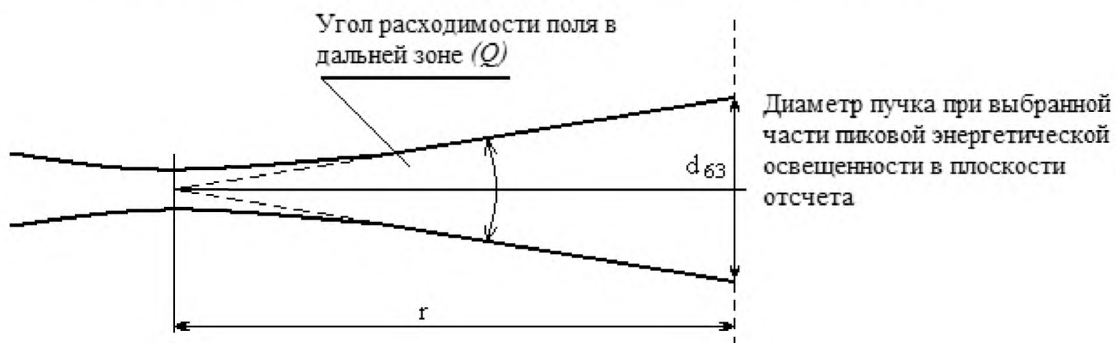
Рисунок 7 – Расположение перетяжки гауссовского пучка
