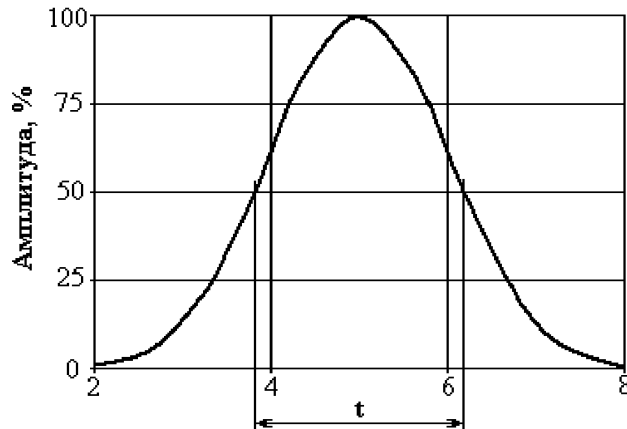
Рисунок 4 – Определение длительности импульса
